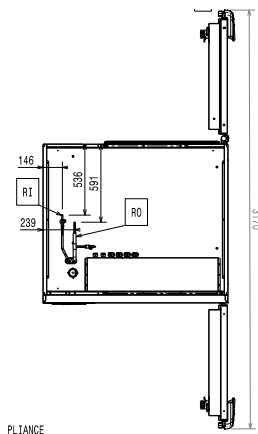
Boven aanzicht
